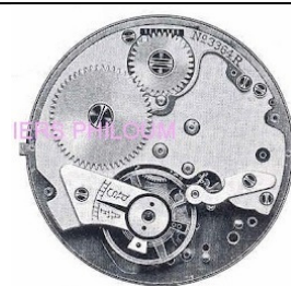
Mouvement Roskopf bonne qualité
